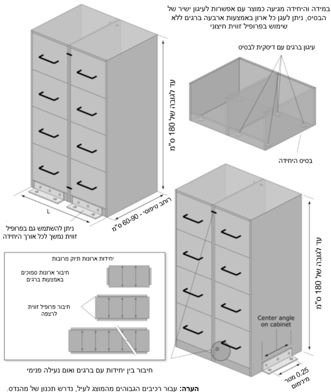
איור 6.5.5.1-5 – עיגון ארונות תיוק לבסיס הרצפה (NE – לא נדרש מהנדס).
