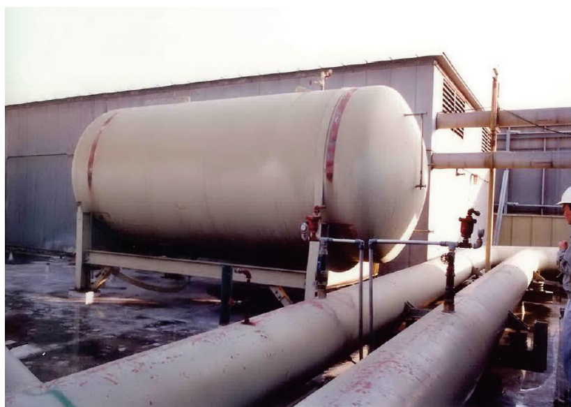
איור 3-6.4.2.1 – מיכל אופקי הנשען על מסגרת בגג בית חולים, אחת מהרצועות נכשלה והמיכל זז כ-15 ס"מ.
