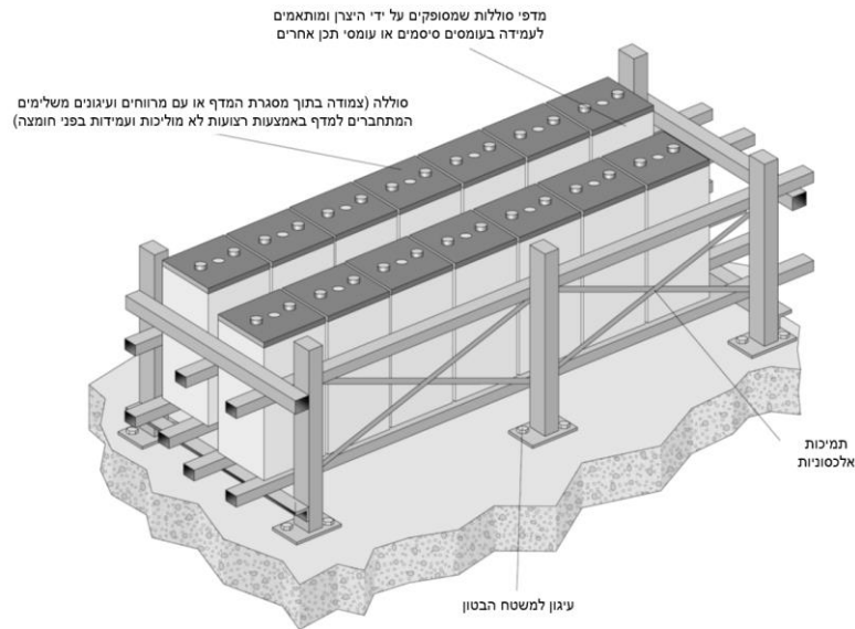
איור 5-6.4.7.4 – סוללות ומדפי סוללות (ER).
