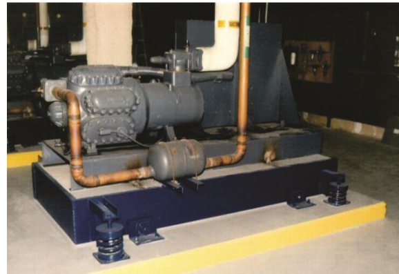
איור 6.4.1.3-6 - קפיצים פתוחים עם סנאברים.
