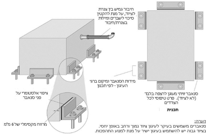
איור 6.4.1.1-7 – פרט עיגון לציוד מונח על הרצפה ומרוסן על ידי סנאברים (ER).
