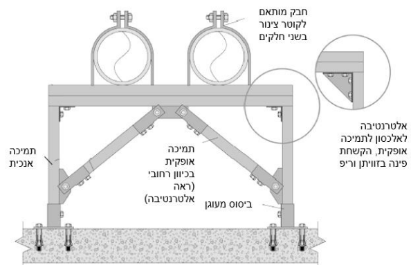
חתך רחבי
