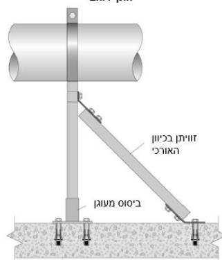
חתך אורכי
