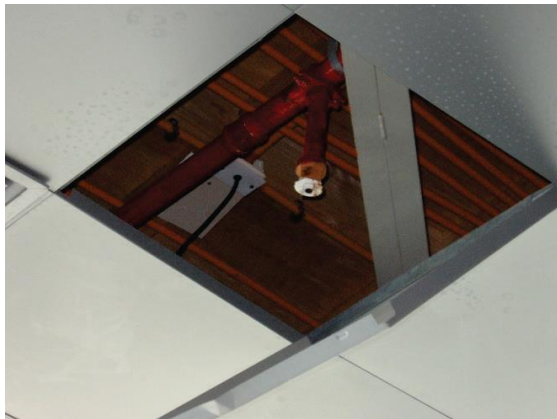
איור 7-6.4.1.1 – דוגמה להתנגשות בין יחידות מתזי המים לסוגים שונים של גימורי תקרה אשר הובילו לנזק בתקרה ובמתלים ולנזקי רטיבות בשדה תעופה.
